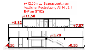
Schnitt S-08 Bauteil C
