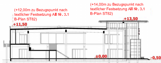
Schnitt S-02 Bauteil A
